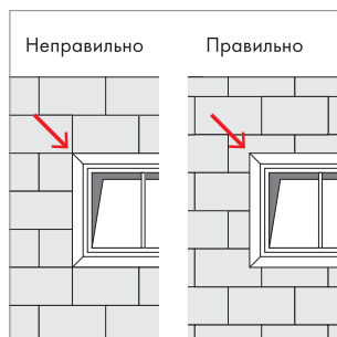
Рис. 23 Схема расположения плит утеплителя на откосах
