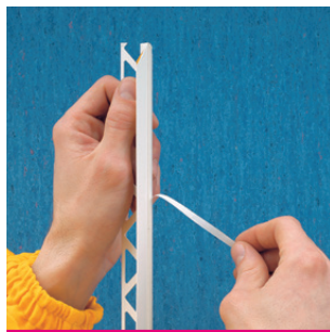
Рис. 26 Установка примыкающего профиля
